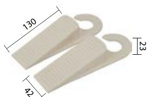
Stavěč dveří 2080 klín (2 ks)
