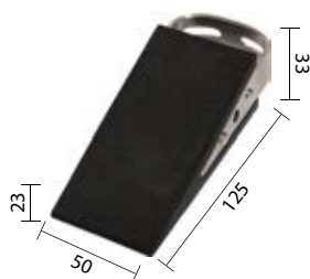
Stavěč dveří podlaha 2060
